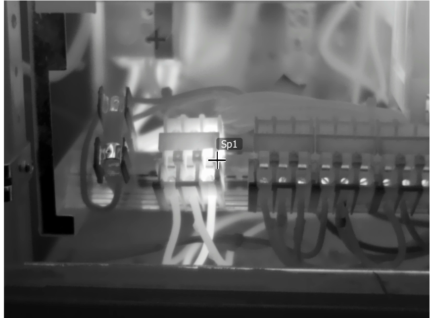
FLIR0013.jpg 2/19/2018 3:54:14 PM
